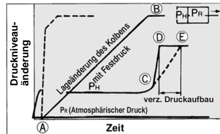
Ausfahrhub beim Start
