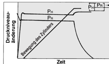
Einfahrhub im normalen Betrieb
