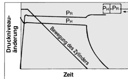
Einfahrhub im normalen Betrieb
