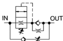
Abluftsteuerung
