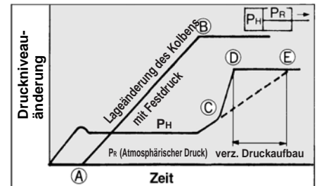
Ausfahrhub beim Start
