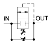
Zuluftsteuerung
