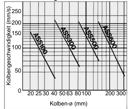
Abluftsteuerung
