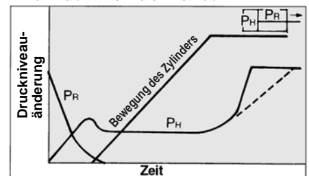
Einfahrhub im normalen Betrieb
