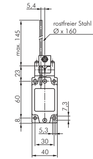
Stangenhebel verstellbar
